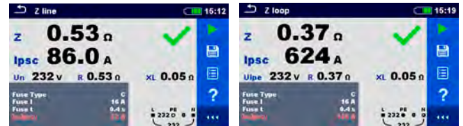
ตัวอย่างการวัดที่ไพลล์ Impedance และ Ipssc ปกติ
