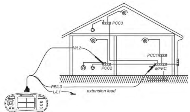
วงจรทดสอบการวัดความต่อเนื่องที่กระแส 200 mA
