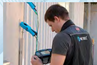
ตรวจวัดความต้านทานดินได้ ทั้งแบบ Clamp และ Ground Rod
