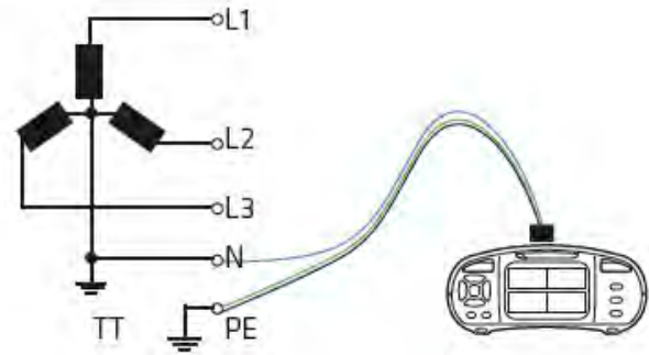
แบบ 2 สาย (ทดสอบที่ได้รับ ระหว่าง N กับ PE)
