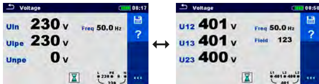
ระดับแรงดันแบบ 1 เฟส
